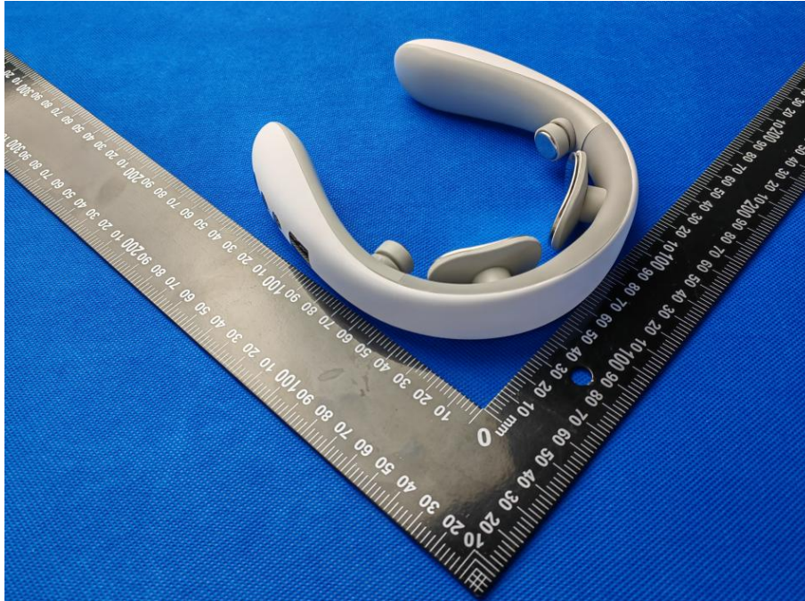
EUT Photo 3
